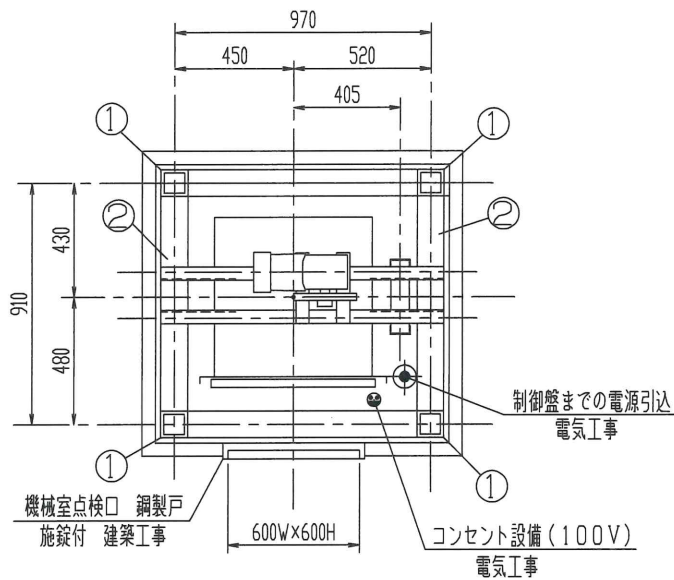
機械室平面図 S = 1 : 20
