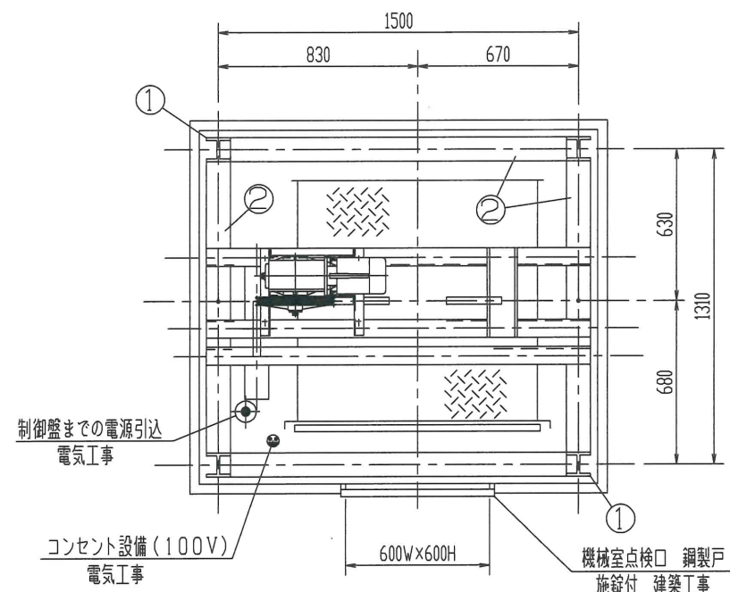
機械室平面図 S = 1 : 20
