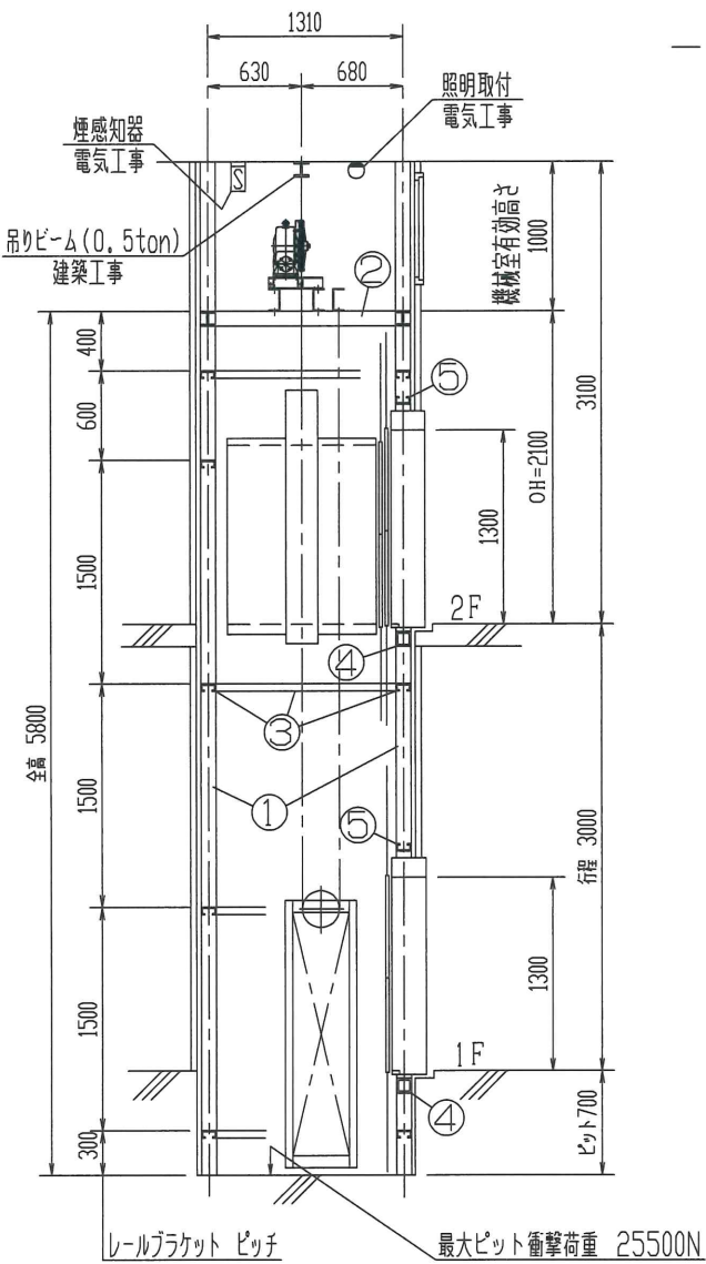
出入口正面鉄骨孔明図及び断面図 S = 1 : 20
