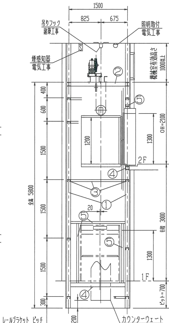
昇降路断面図 S = 1 : 4 0 (A-A矢視)
