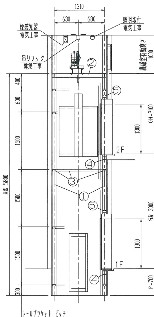
昇降路断面図 S = 1 : 40
