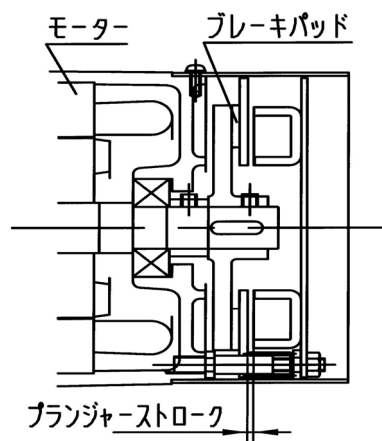
ディスクブレーキ方式 (TDM型)
