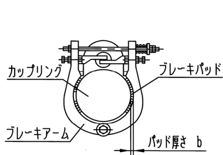
(図2:ドラムブレーキ方式)
