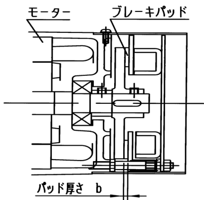
(図1:ディスクブレーキ方式)
